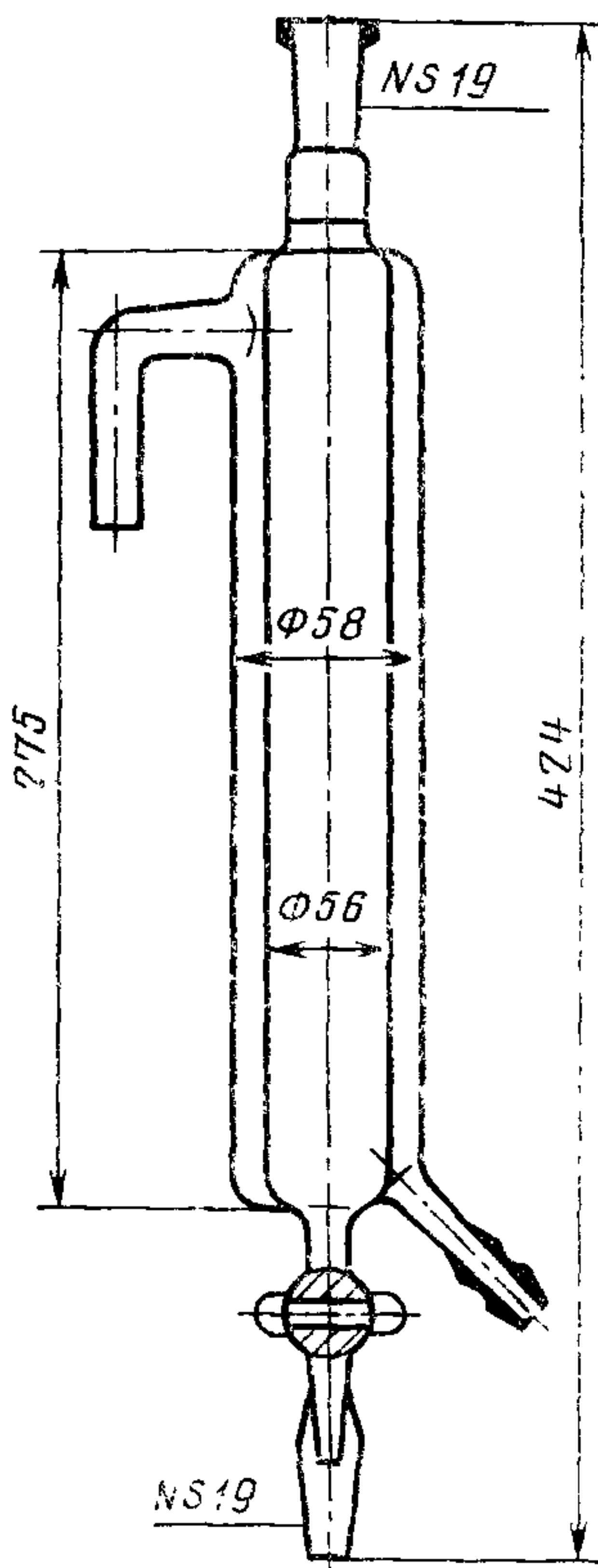
Делительная воронка с рубашкой для термостатирования
